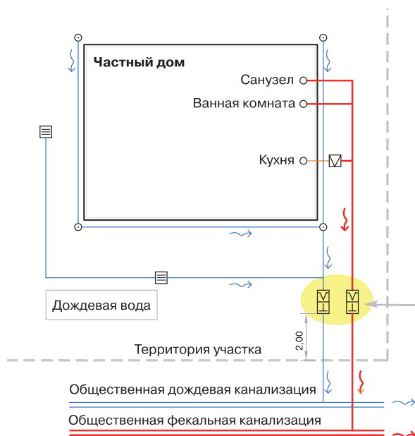
Рис. 1 - Частный дом
