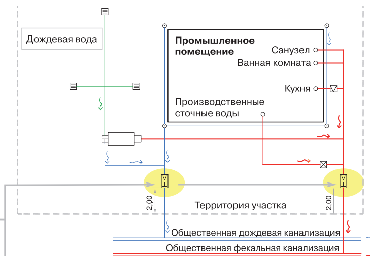
Рис. 2 - Промышленное помещение
