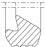
Сечение уплотнителя
