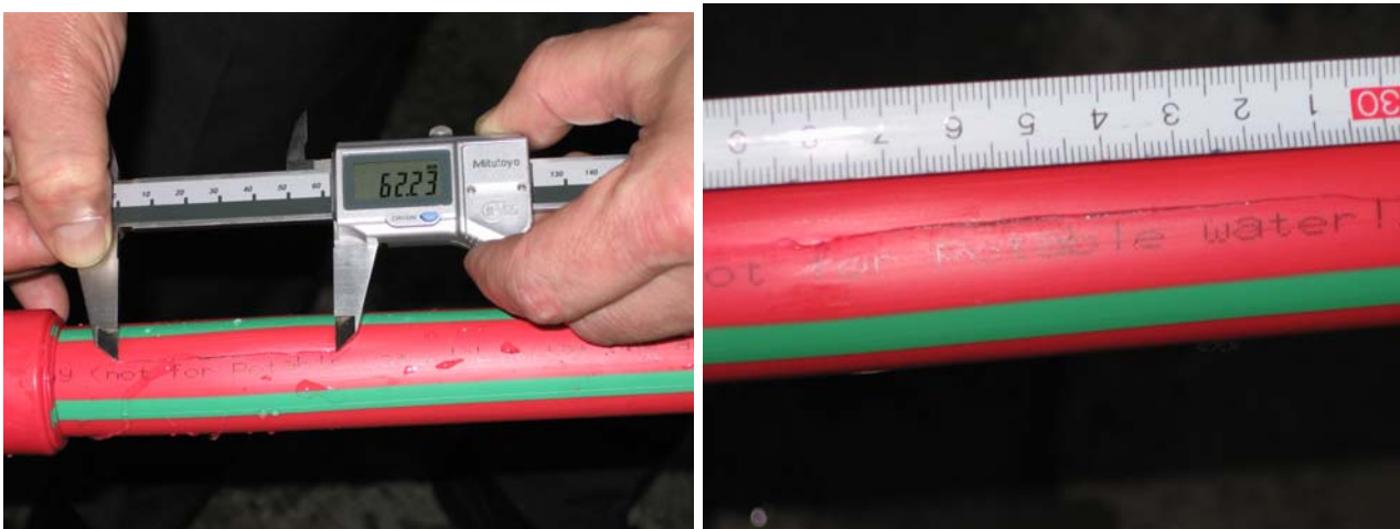
Рисунок ПД2 – Характер разрушения трубопроводов
