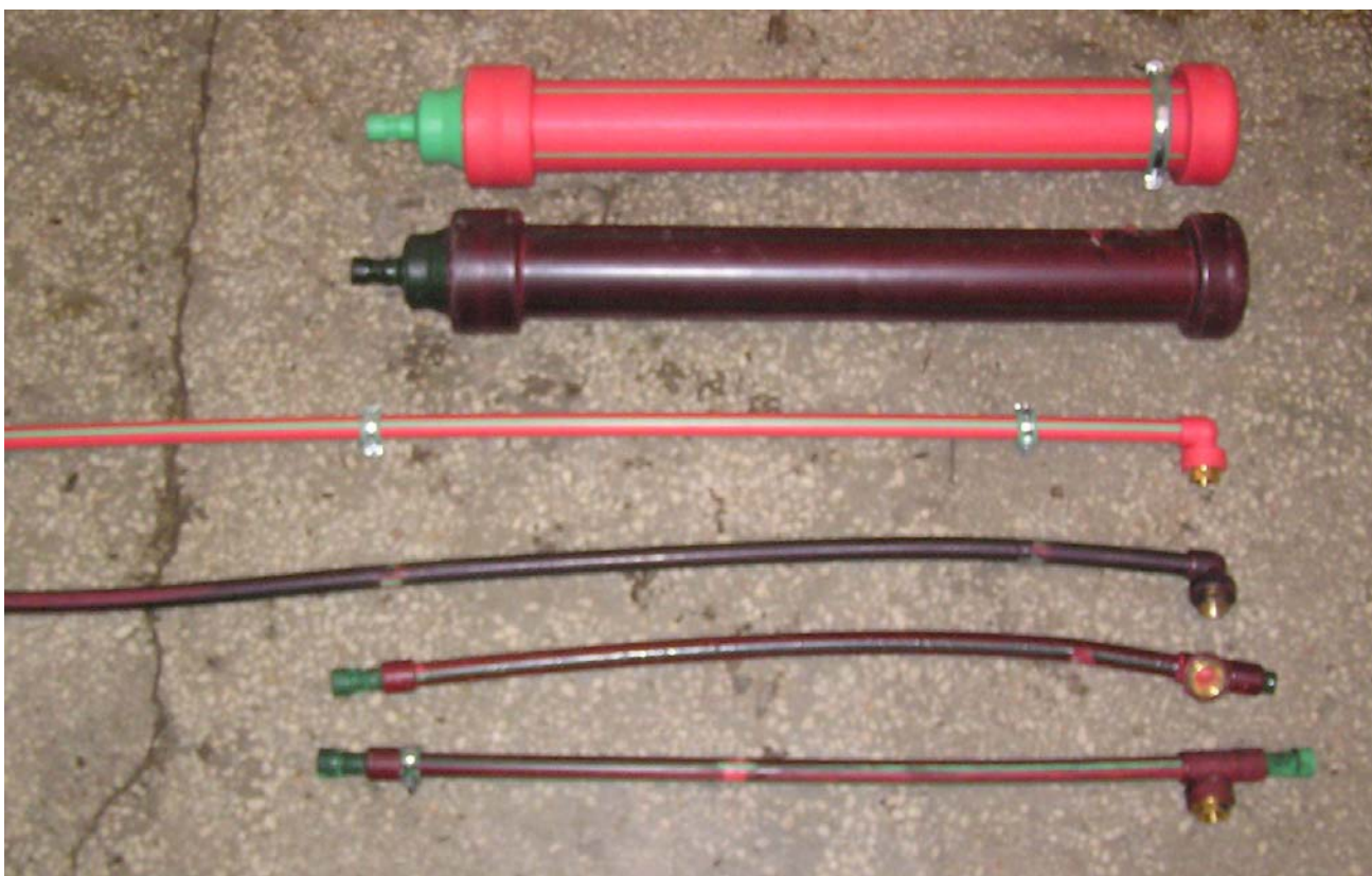
Рисунок ПД4 – Состояние труб до и после испытаний
